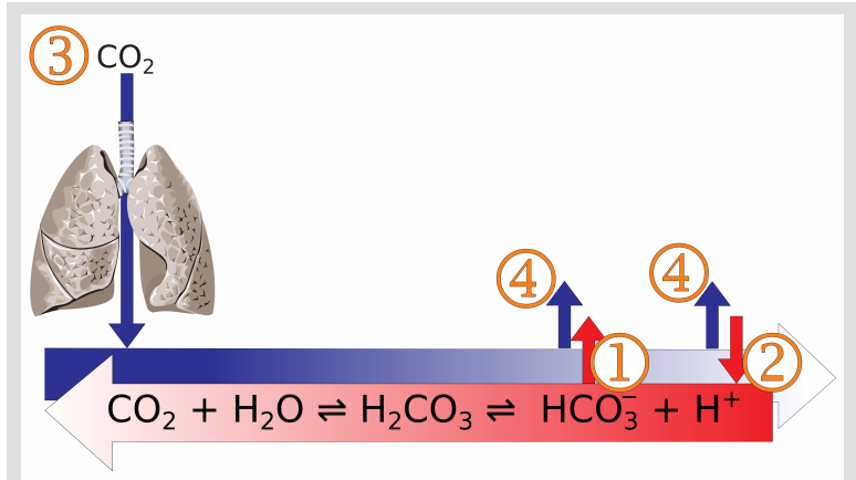
Figura 28.4. Aumento del bicarbonato
