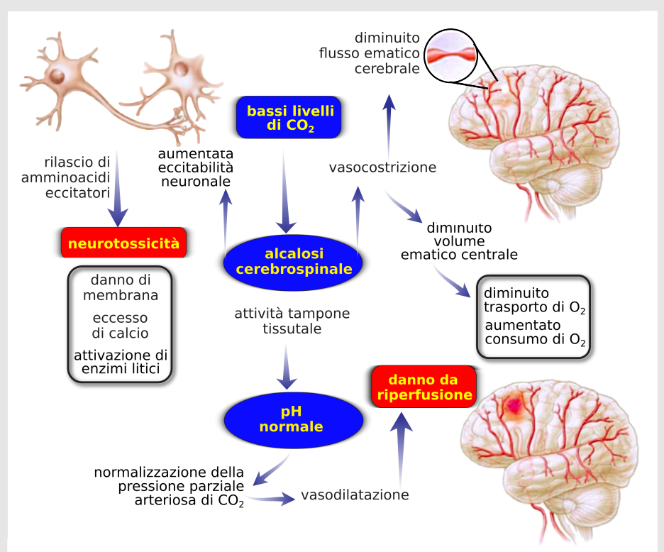
Figura 28.13. Effetti neurologici dell'ipo-capnia. Da: Laffey (2002), modificato e ridisegnato
