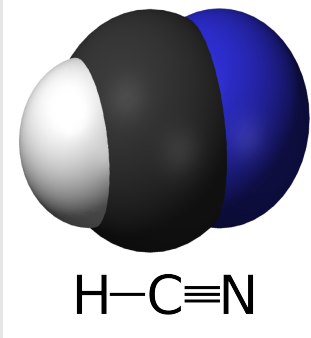
Figura 39.13. Acido cianidrico, struttura
