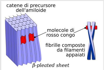
Figura 6.22. Amiloide: struttura.
