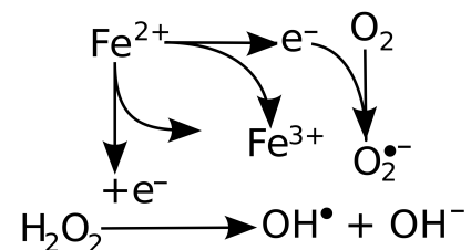
Figura 6.2. Reazione di Fenton
