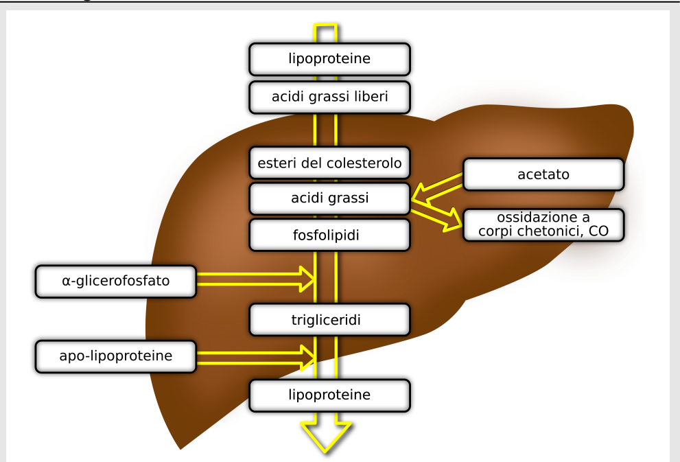
Figura 6.10. Schema sintetico del metabolismo degli acidi grassi nel fegato
