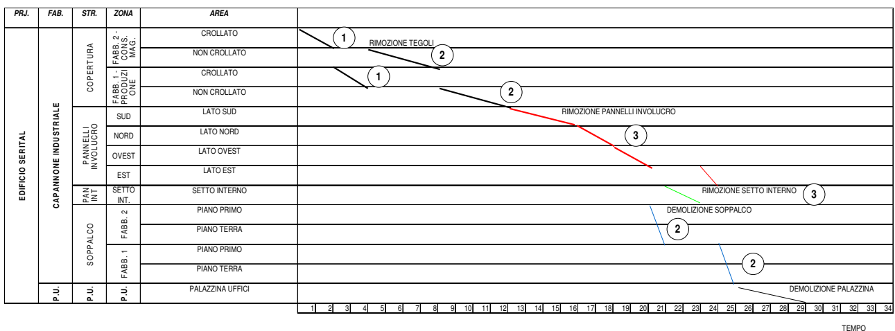
Figura 7: programma delle demolizioni con il diagramma flow-line con rischi fondamentali
