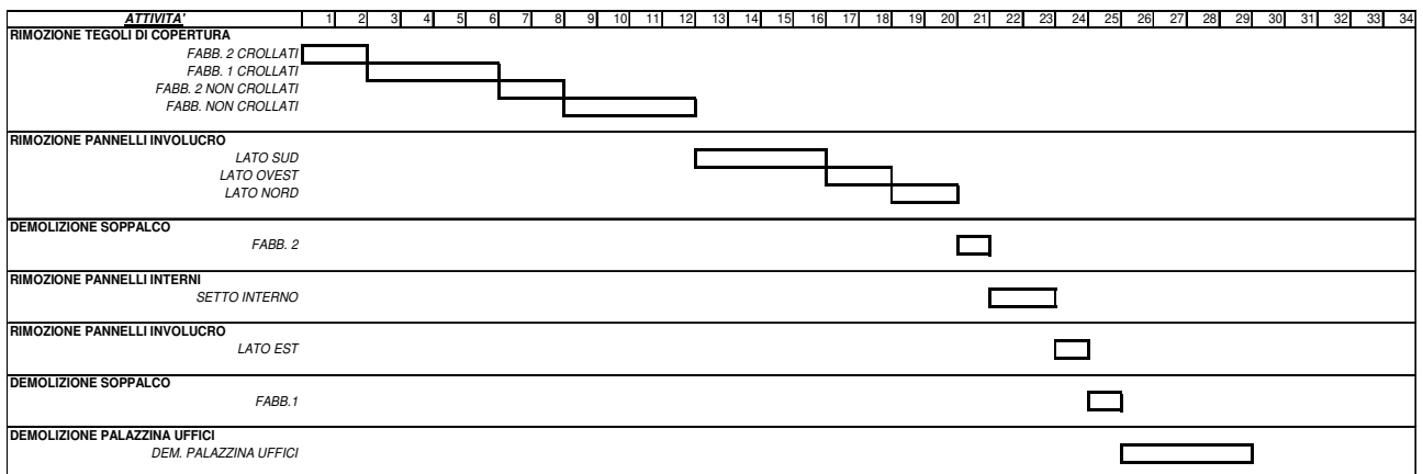
Figura 6: diagramma di Gantt per la fase di demolizione
