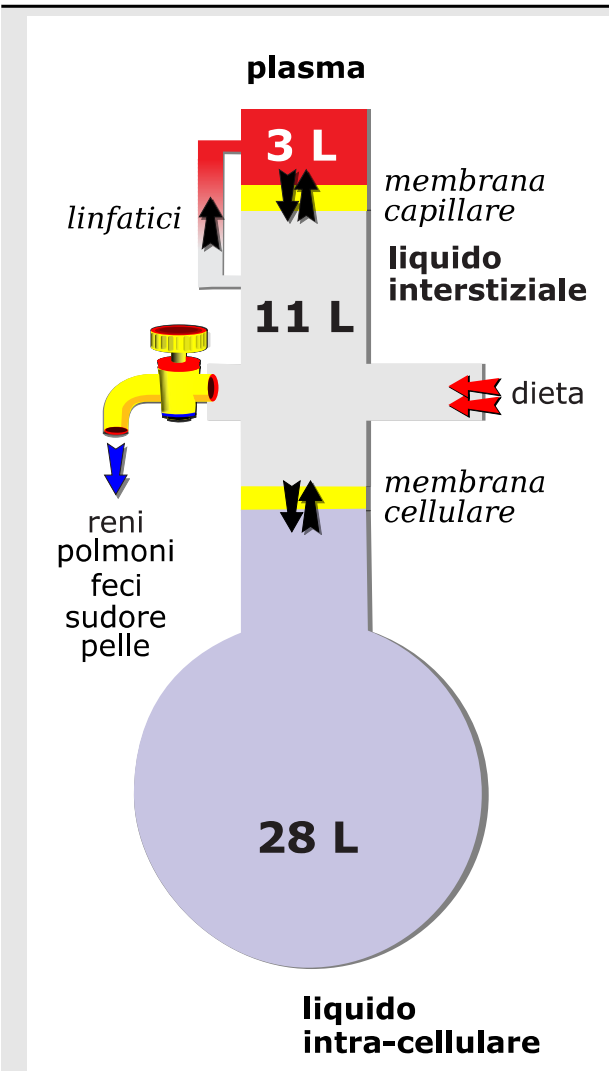
Figura 1.7. Liquidi: compartimenti
