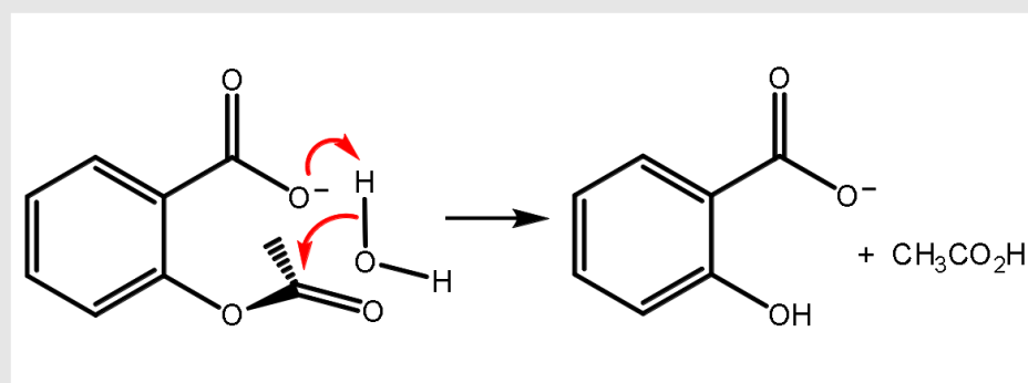
Figura 42.1. Idrolisi dell'aspirina
