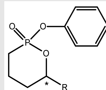
Figura 42.19. Estere fosfonato ciclico (dx.)
