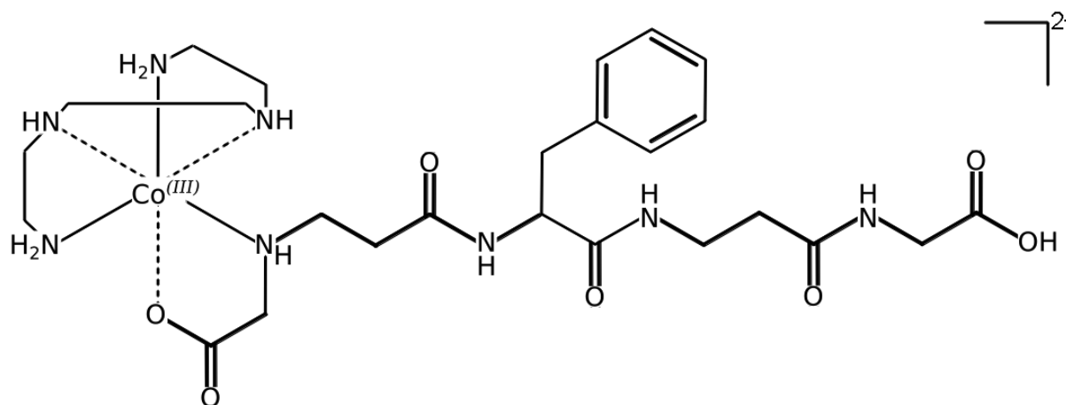
Figura 42.28. Complesso trienico di Co (III) inerte
