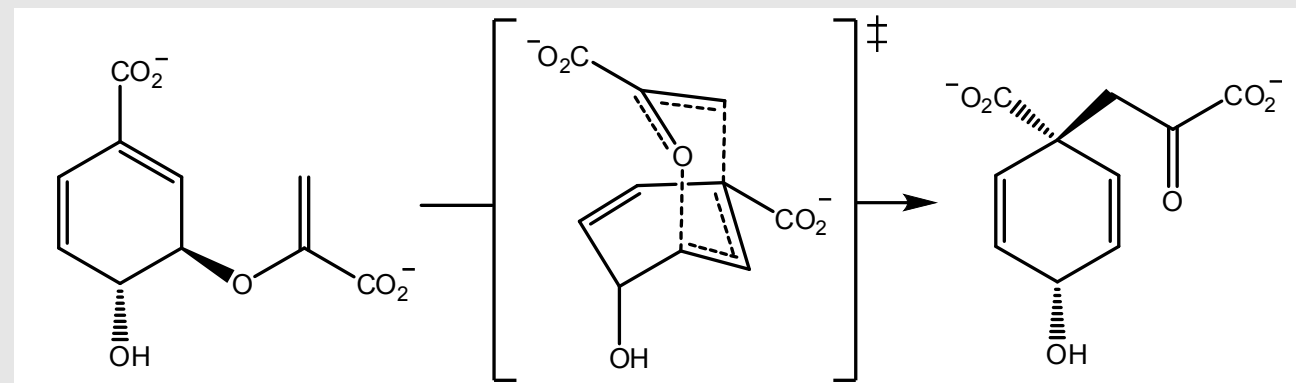
Figura 42.15. Trasposizione o riarrangiamento di Claisen
