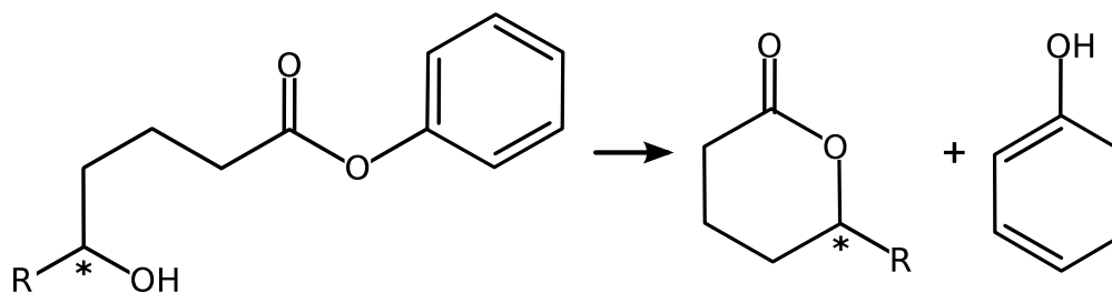
Figura 42.21. Reazione di rottura
