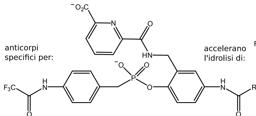
Figura 42.11. Coppie di antigeni e relativi substrati
