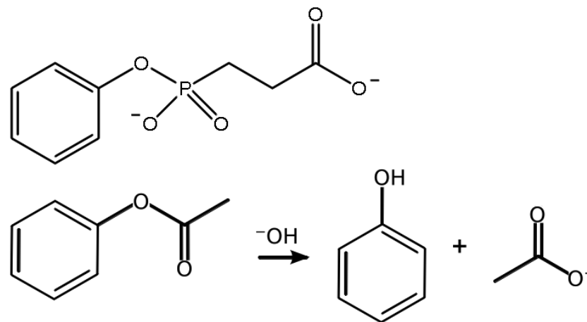
Figura 42.12. Reazione con un substrato idrofobica
