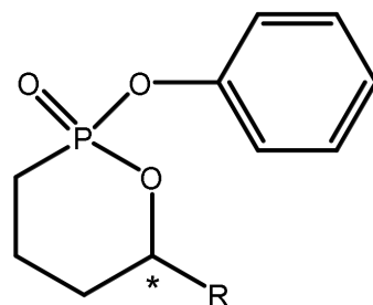
Figura 42.23. Estere fosfonato ciclico usato come aptene nella produzione di anticorpo, che è risultato un inibitore competitivo delle reazioni catalizzate dall'anticorpo stesso, dimostrando che la catalisi avviene nel sito di legame dell'estere fosfonato/inibitore
