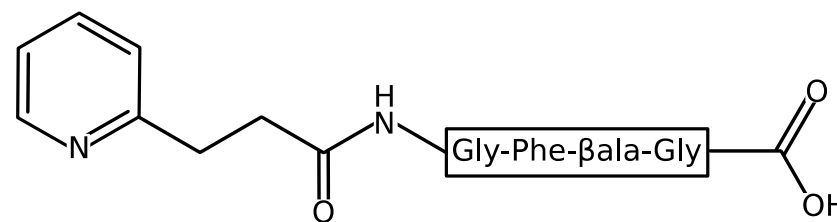
Figura 42.29. Peptide
