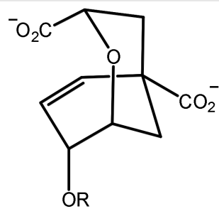
Figura 42.16. Diacido biciclico (in alto)
