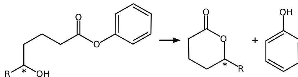
Figura 42.20. Reazione di ciclizzazione a sei atomi
