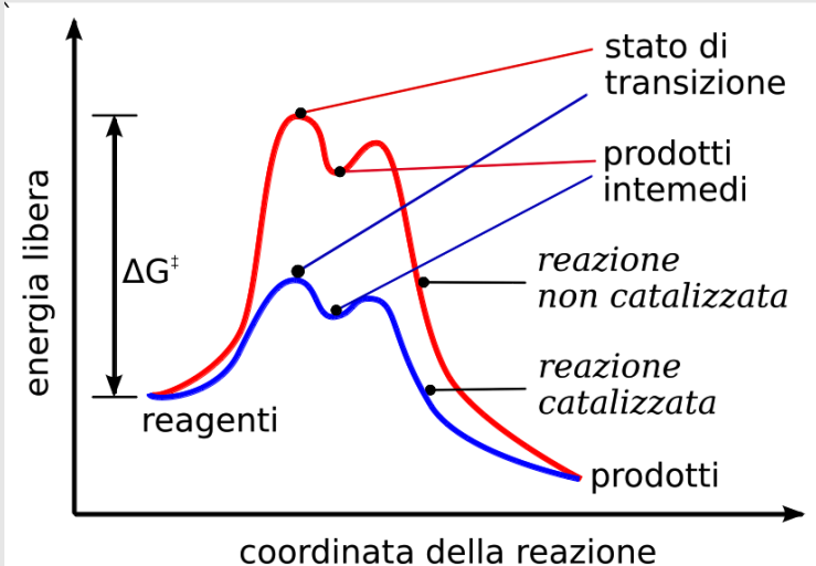
Figura 42.6. Stato di transizione
