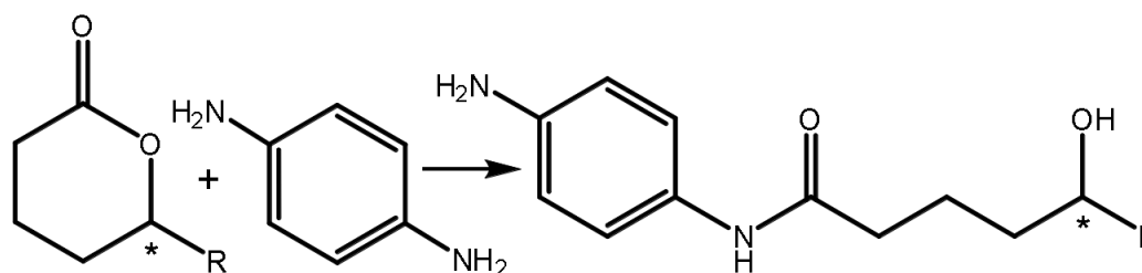
Figura 42.22. formazione di un legame ammidico bi- molecolare
