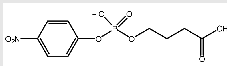
Figura 42.10. Analogo stabile di struttura di transizione tetraedrica
