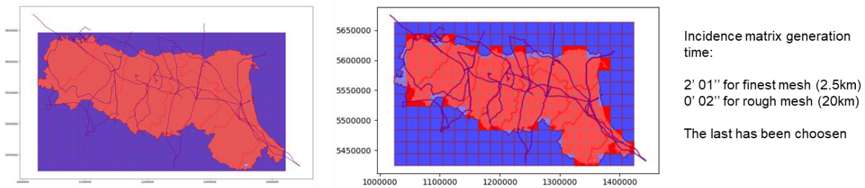
Figura 29. Risultato del processo di realizzazione della mesh adottando due diverse dimensioni della griglia di calcolo.
