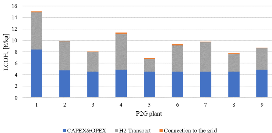
Figura 35. LCOH atteso.
