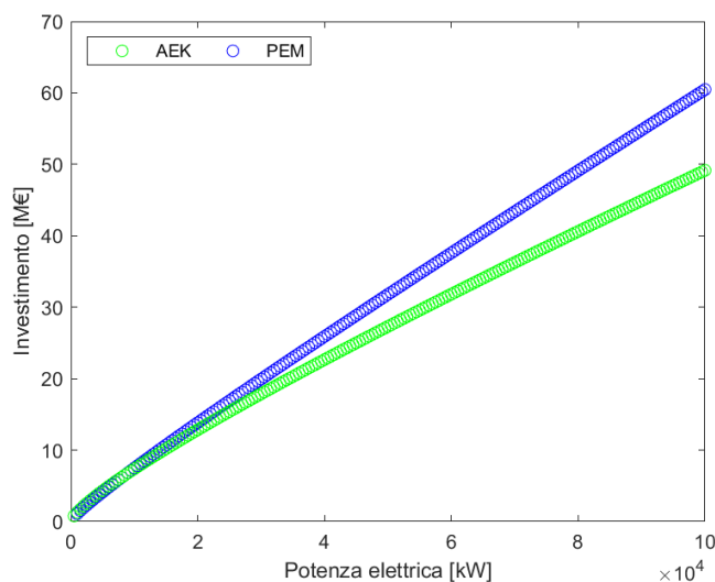
Figura 14. Costo di investimento elettrolizzatori alcalini e PEM.
