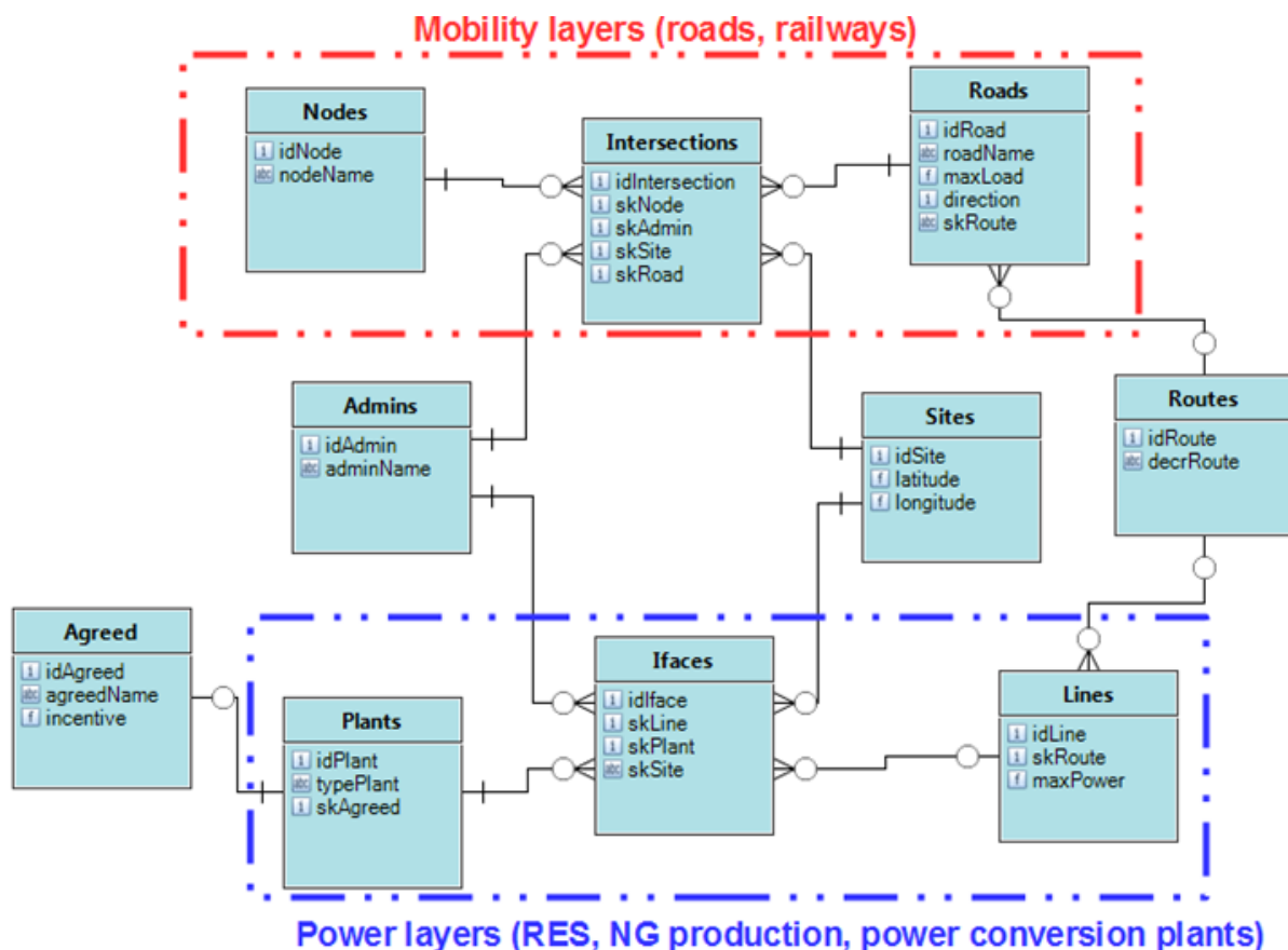
Figura 21. Struttura del database realizzato.
