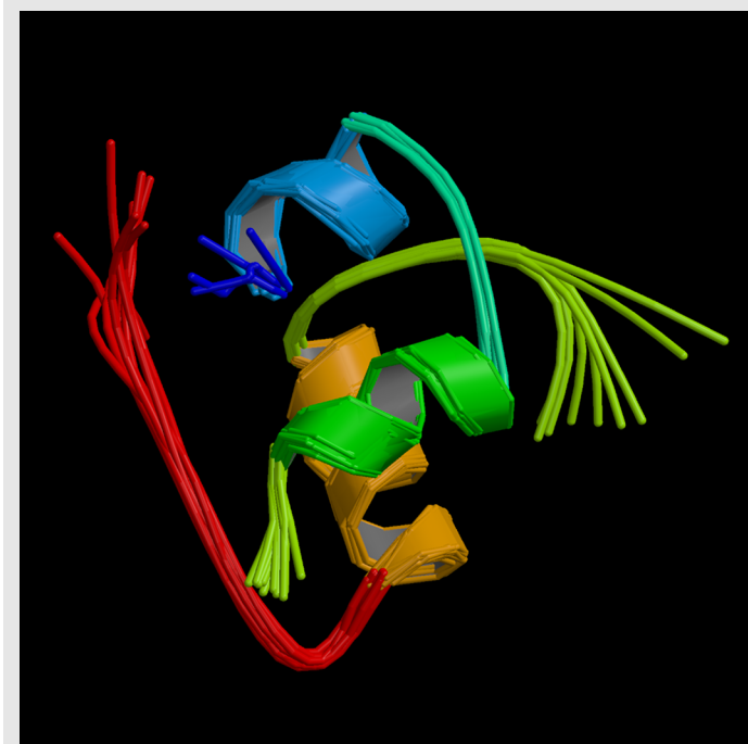
Figura 35.11. Struttura 3D dell'insulina Rendering di 1g7a.pdb (Bohem, 1999) ottenuto con molscript (Kraulis, 1991) e Raster3D (Merrit, 1997)
