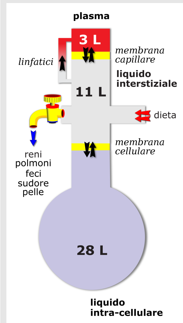
Figura 1.7. Compartimenti liquidi
