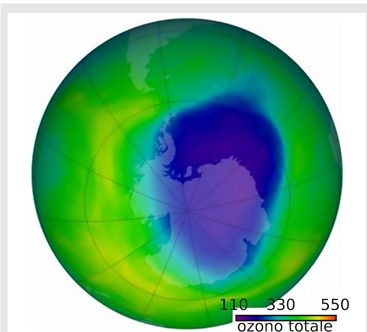
Figura 2.4. Buco dell'ozono. Modificata da wildweather.com/forecastblog
