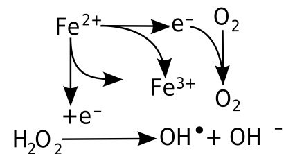
Figura 6.2. Reazione di Fenton
