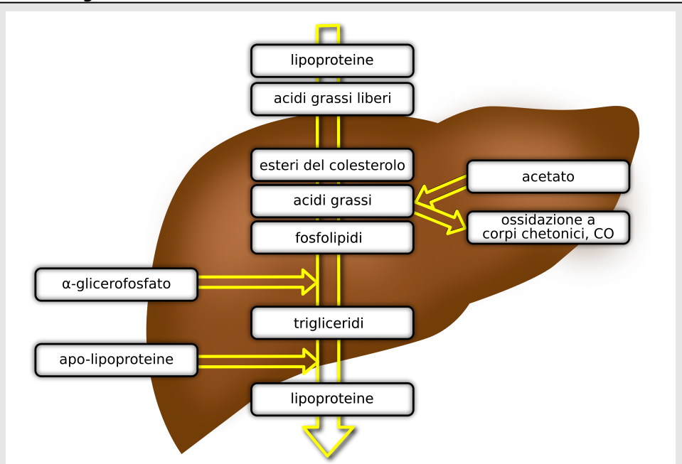
Figura 6.9. Schema sintetico del metabolismo degli acidi grassi nel fegato
