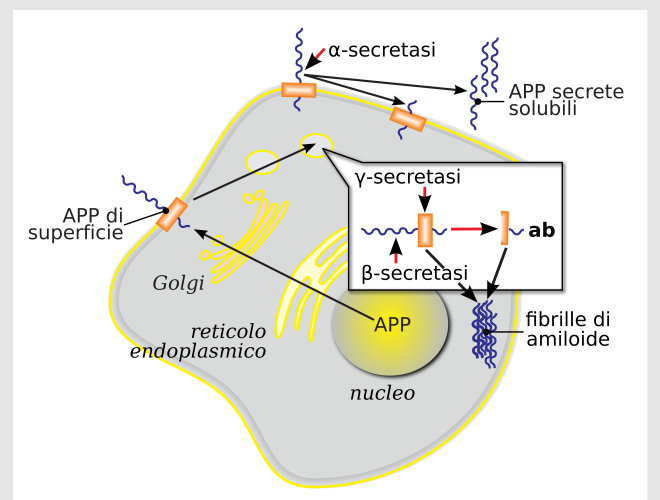
Figura 6.18. Precursori dell'amiloide. APP: amiloid precursor protein (precursore della proteina amiloide)
