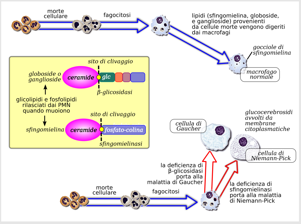
Figura 6.13. Malattie di Niemann-Pick e Gaucher: patogenesi. Da: AA vari (1998)
