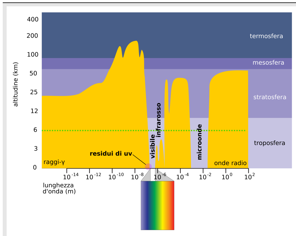
Figura 20.1. Capacità di penetrazione delle radiazioni attraverso l'atmosfera terrestre
