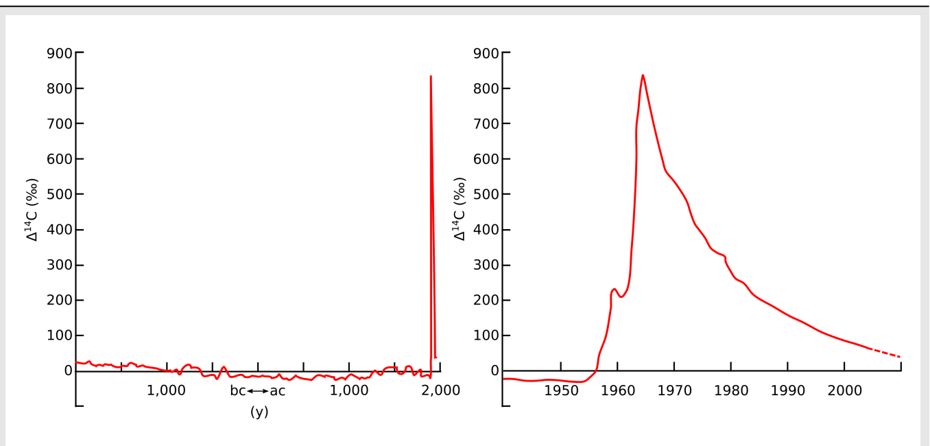
Figura 20.2. Livelli di ^{14}C nella biomassa. Dati originali da Levin (2004) e Stuiver (1977). bc: prima di Cristo; ac: dopo Cristo
