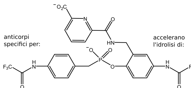
Figura 42.11. Coppie di antigeni e relativi substrati
