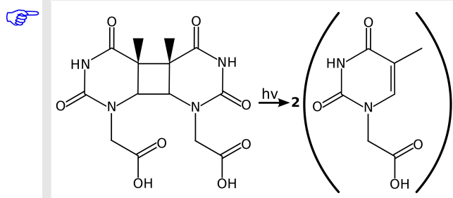
Figura 42.5. Ciclo-reversione da dimero di timina a 2 timine
