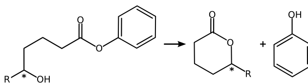
Figura 42.20. Reazione di ciclizzazione a sei atomi
