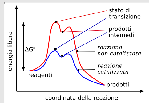
Figura 42.6. Stato di transizione
