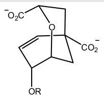
Figura 42.16. Diacido biciclico (in alto)
