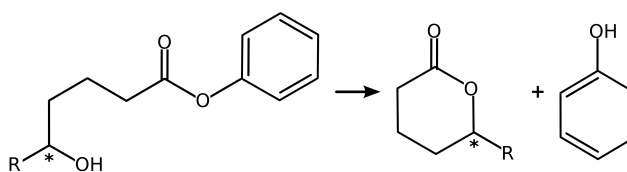
Figura 42.21. Reazione di rottura
