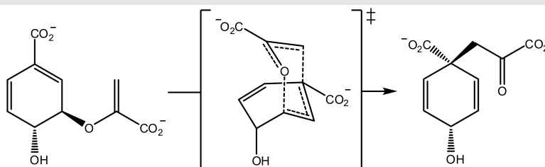
Figura 42.15. Trasposizione o riarrangiamento di Claisen
