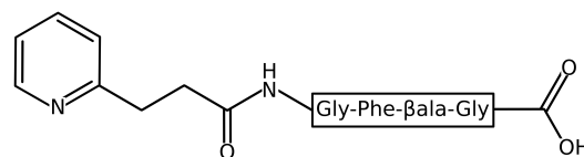
Figura 42.29. Peptide
