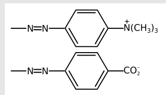
Figura 42.2. p -azobenzene-trimetilammonio (in alto); p -azobenzoato (in basso)
