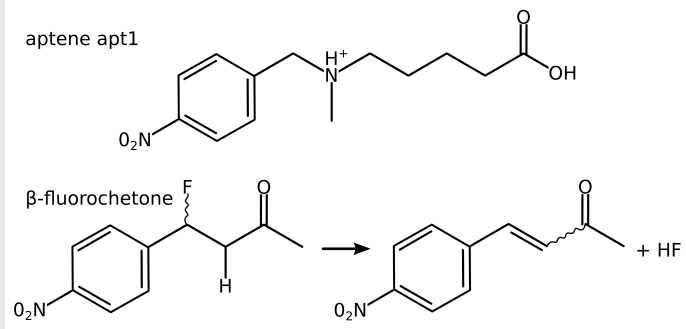
Figura 42.3. Aptene apt1 (sopra); reazione di eliminazione di HF da \beta -fluorochetone
