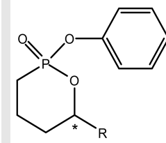
Figura 42.19. Estere fosfonato ciclico (dx.)
