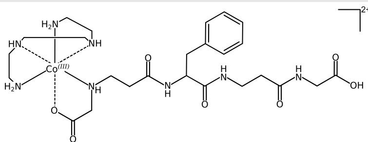
Figura 42.28. Complesso trienico di Co (III) inerte
