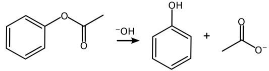
Figura 42.12. Reazione con un substrato idrofobica
