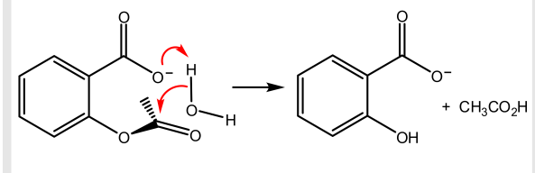
Figura 42.1. Idrolisi dell'aspirina
