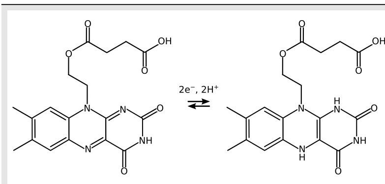
Figura 42.27. I tre anelli sono complanari nella forma ossidata di flavina (a sinistra)
