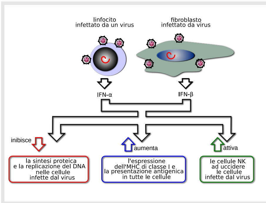
Figura 17.10. Interferoni
