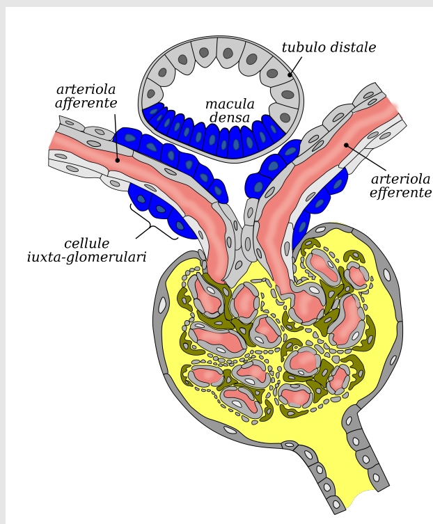
Figura 26.5. Schema anatomico di reni e surrenali
