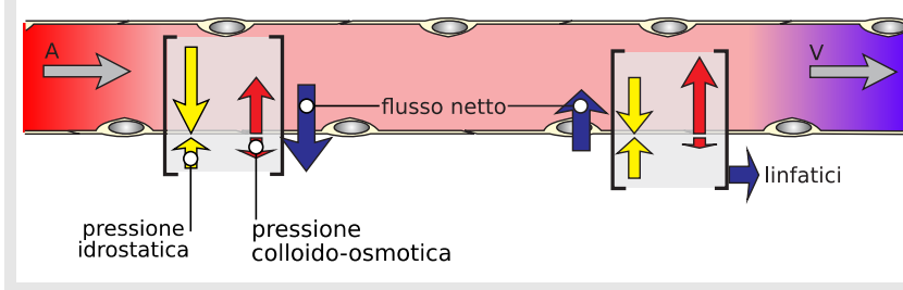
Figura 26.8. Formazione del trasudato: scambio di fluidi a livello capillare
