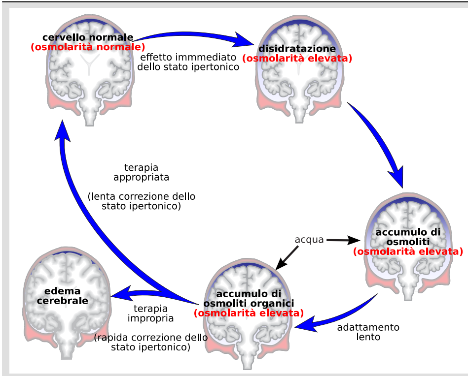
Figura 26.18. Effetti dell'iper-natriemia sul cervello ed adattamento
