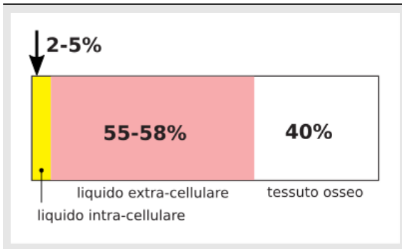
Figura 26.9. Distribuzione del sodio
