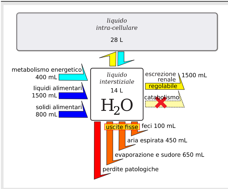
Figura 26.3. Bilancio di ingressi e uscite dell'acqua. Valori riferiti a condizioni standard di temperatura e umidità per un soggetto normale a riposo Il ricambio giornaliero di acqua è complessivamente del 8-9%
