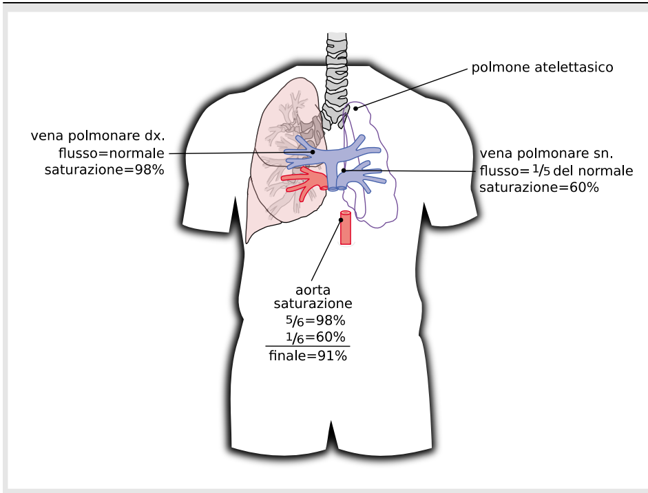
Figura 39.2. Alterazione del rapporto ventilazione/perfusione nell'atelettasia del polmone di sn.
